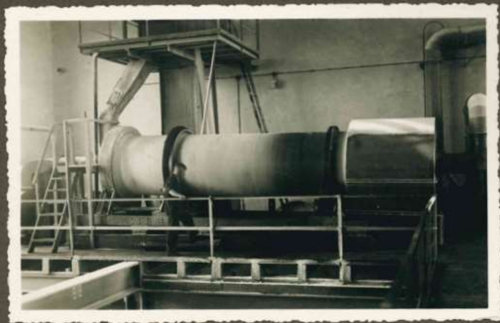
Ģranulatorā cukuru žāvē un sadala pēc rupjuma.
