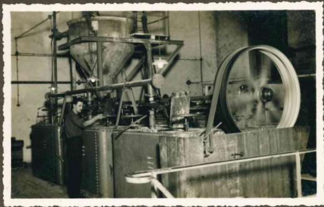
Sulas kaļķotavā ar kaļķu pienu sajauc cukuru saturošu sulu.
