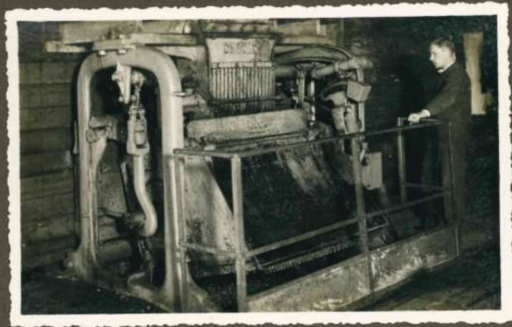
Automatiskos svaros c.bietes sver un svaru reģistrē.
